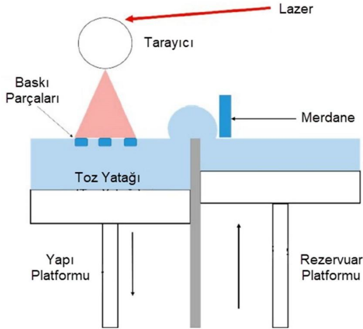
Şekil 7. SLS yönteminin şematik gösterimi (Gueche ve diğerleri, 2021).
