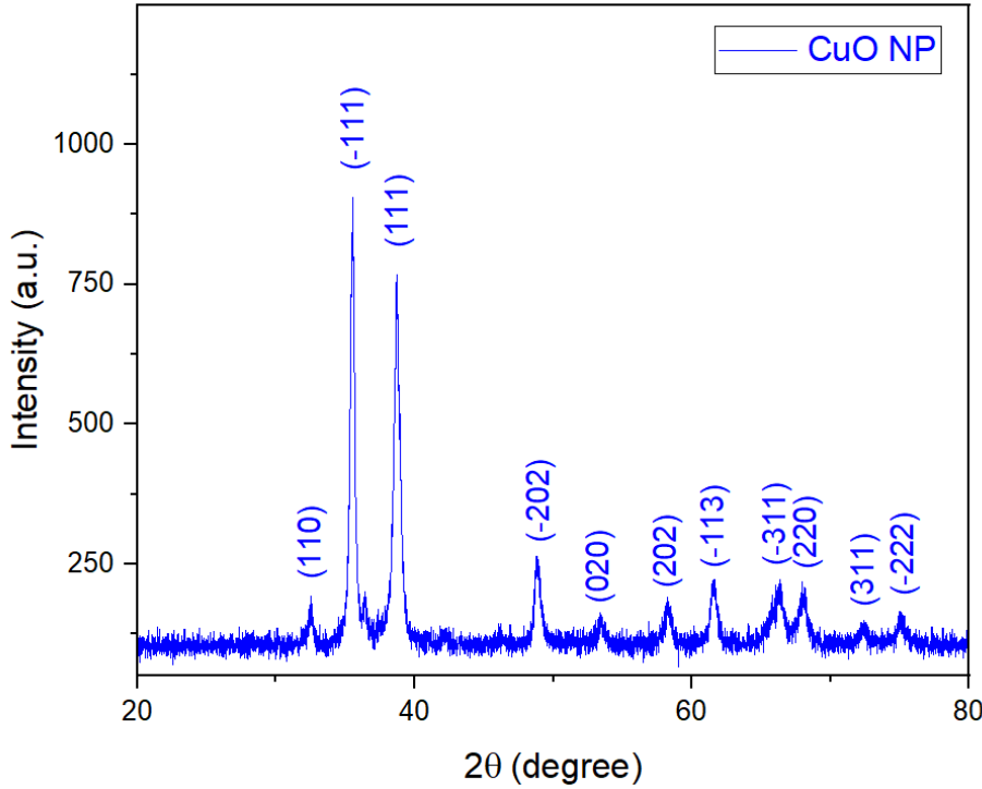
Şekil 1. CuO NP'lerin XRD deseni
