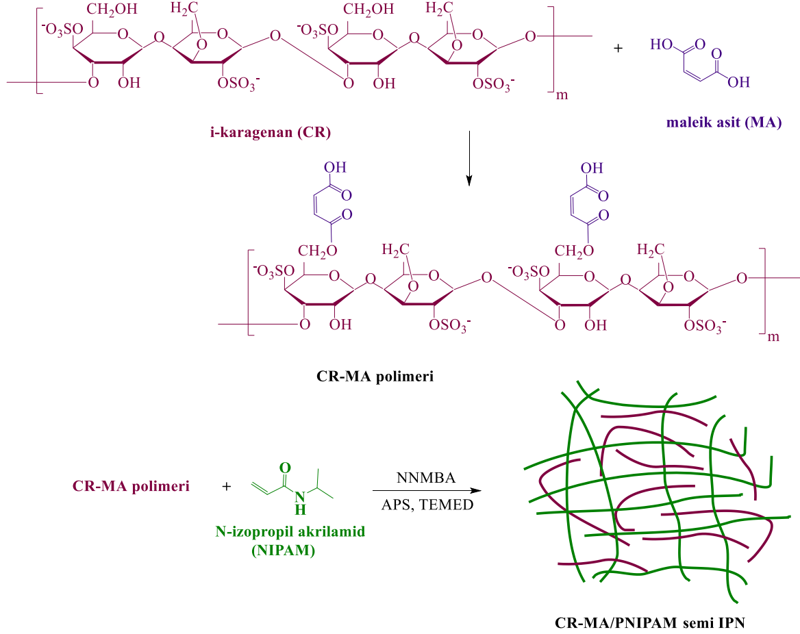
Şekil 1. Hazırlanan CR-MA/PNIPAM hidrojelinin olası polimerleşme mekanizması.
